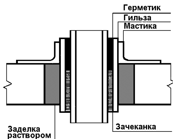
Рис. 8. Герметизация стыка (технологического шва) между железобетонными плитами радонозащитного барьера
