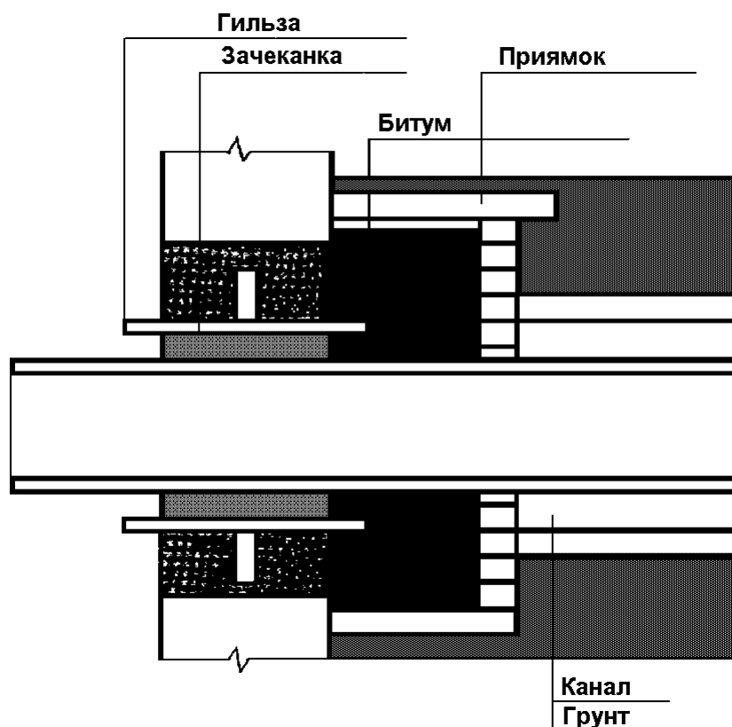
Рис. 10. Герметизация узла ввода-вывода трубопровода в здание
