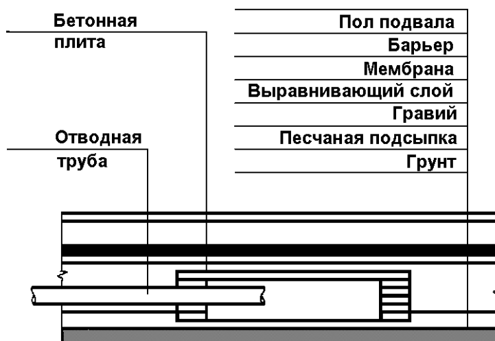
Рис. 7. Камера для сбора радона
