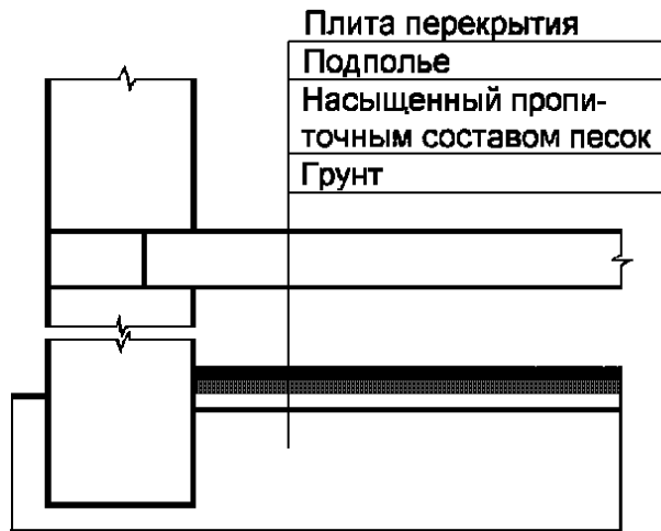
Рис. 2. Пропиточная противорадионовая изоляция грунтового пола подполья
