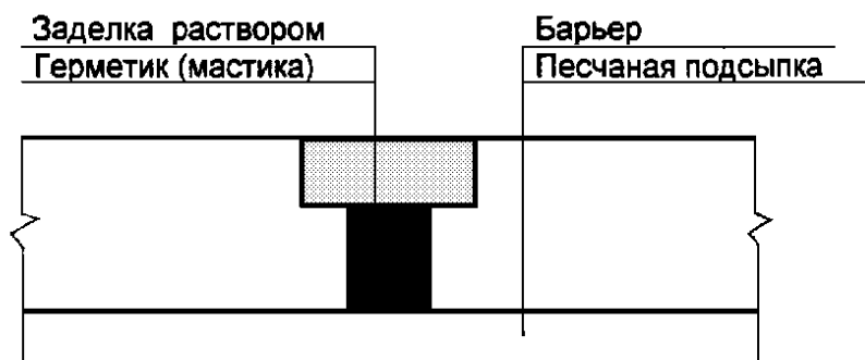
Рис. 8. Герметизация стыка (технологического шва) между железобетонными плитами радонозащитного барьера
