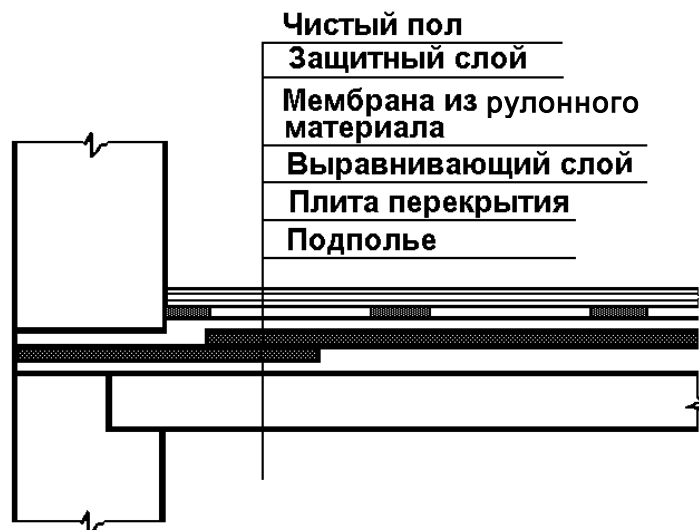
Рис. 4. Радоноизолирующая мембрана в подвальном перекрытии
