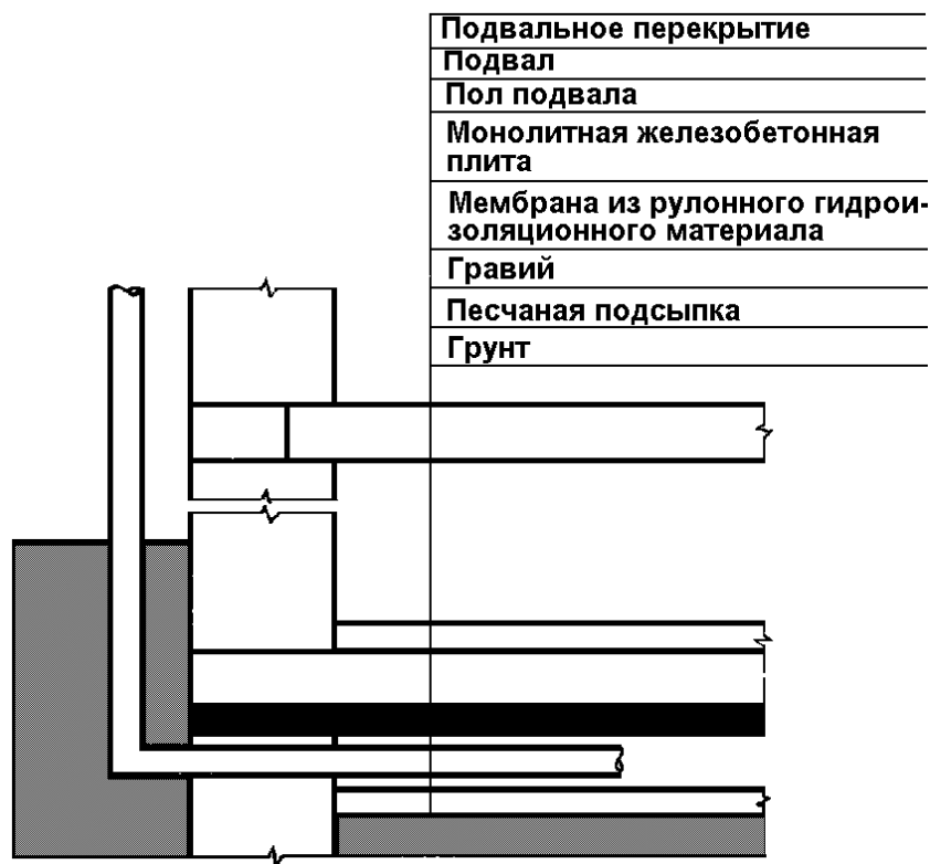
Рис. 6. Коллектор радона, мембрана, барьер
